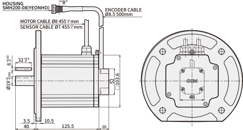
K20BK750NC-E (Encoder type) Weight : 5.4Kg
