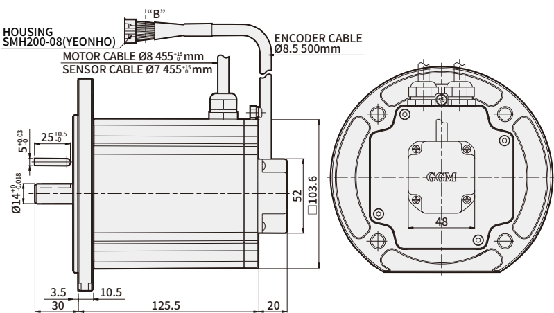
K16BK750NC-E (Encoder type) Weight : 5.1Kg
