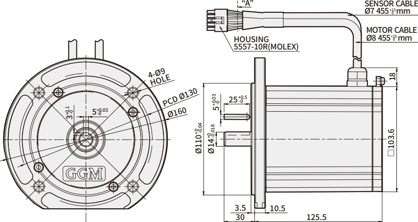
K16BK750NC Weight : 5Kg
