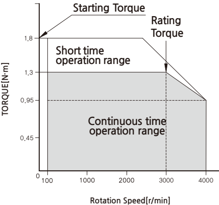
K10FS400NC / K10FH400NC
