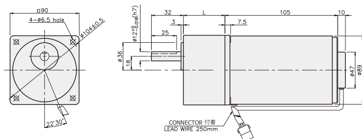
K9RG40N□-SU + K9G□B(C)
